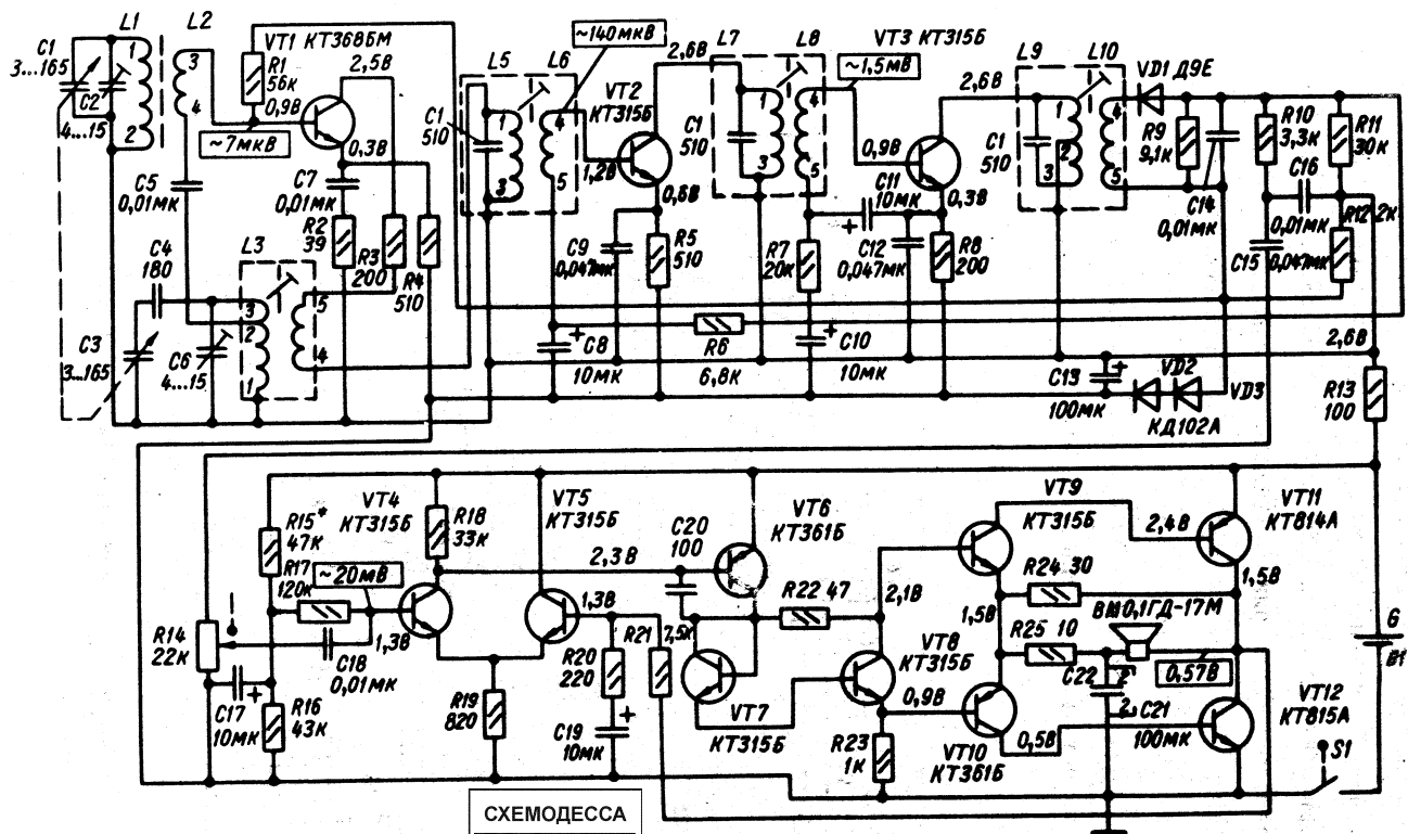
Принципиальная электрическая схема приемника "ВОЛХОВА"
