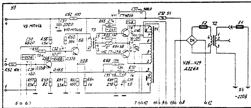
Усилитель мощности
