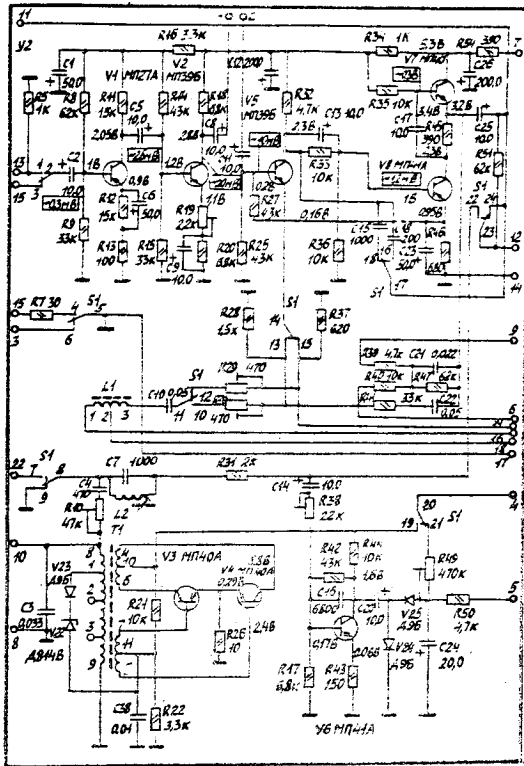
Блок предварительного усилителя с генератором записи
