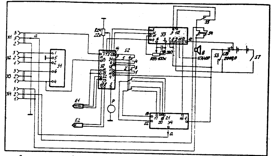
Структурная схема магнитофона „Ритм-301“
