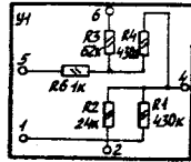
Блок делителей напряжения
