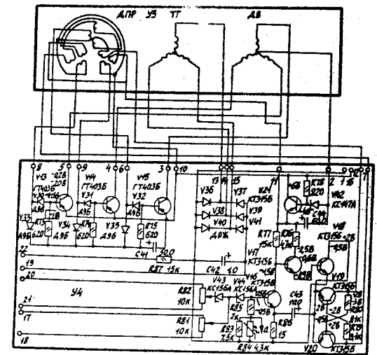
Блок коммутатора двигателя
