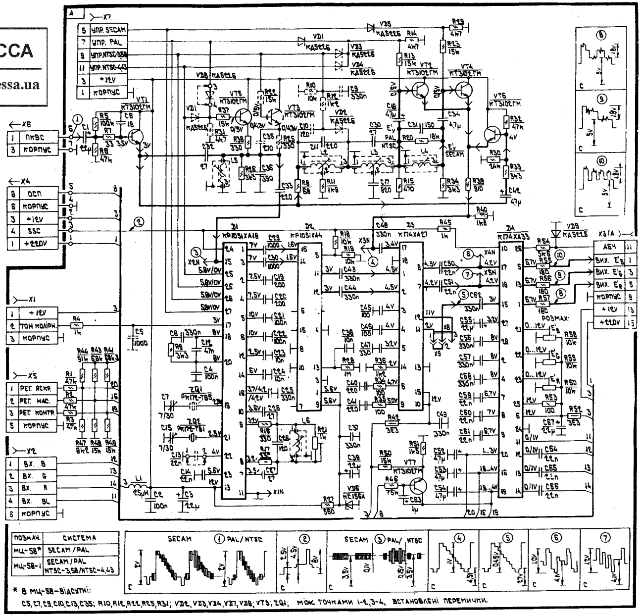
Схема электрическая функциональная МЦ-58, МЦ-58-1
