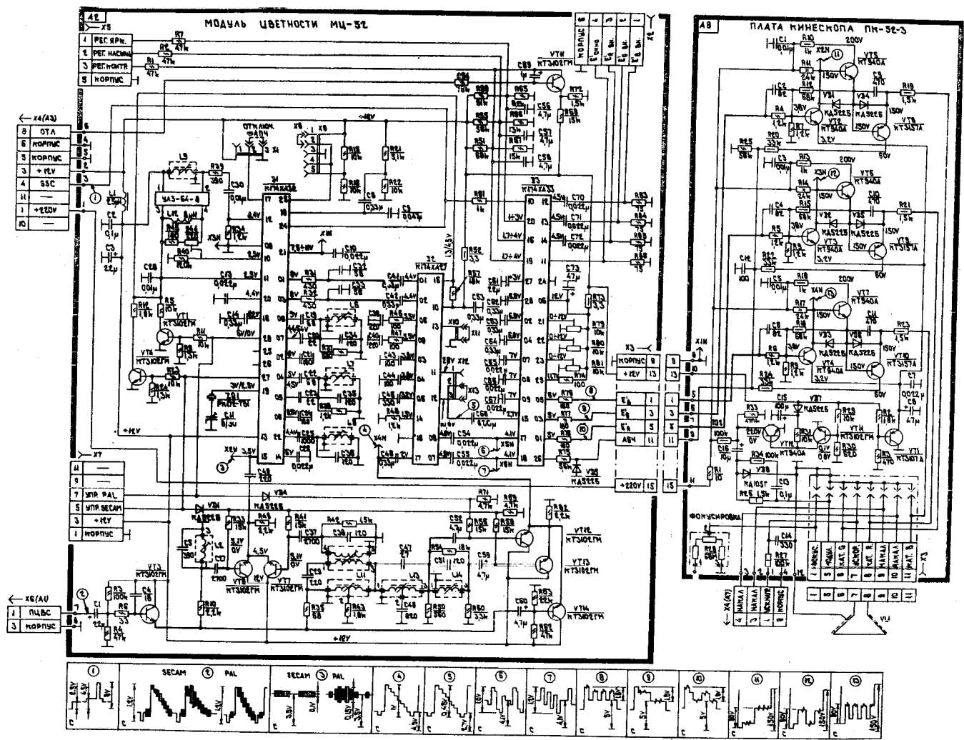
Модули цветности МЦ-52, ПК-52-3
