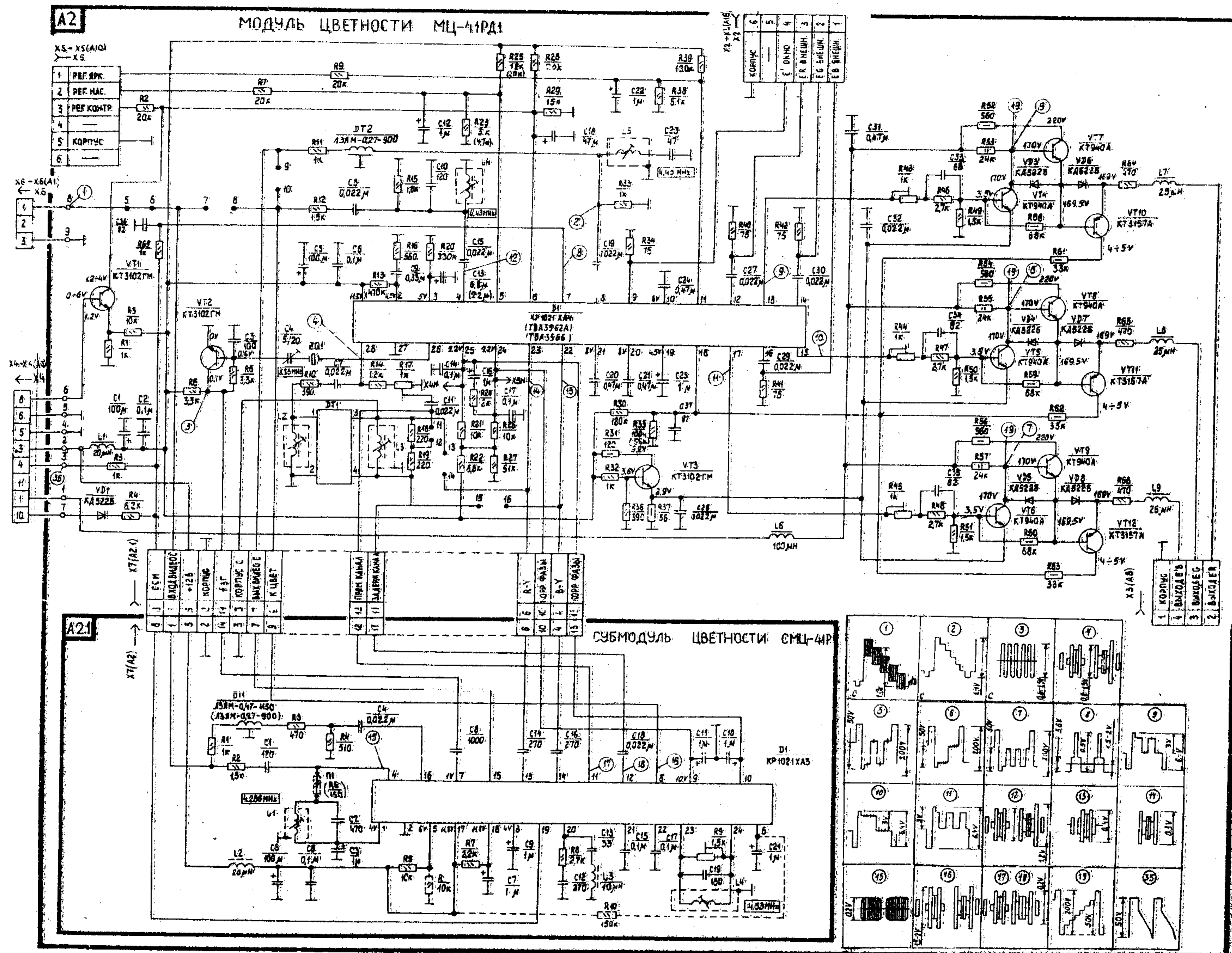
Модули цветности МЦ - 41РД1, СМЦ - 41Р
