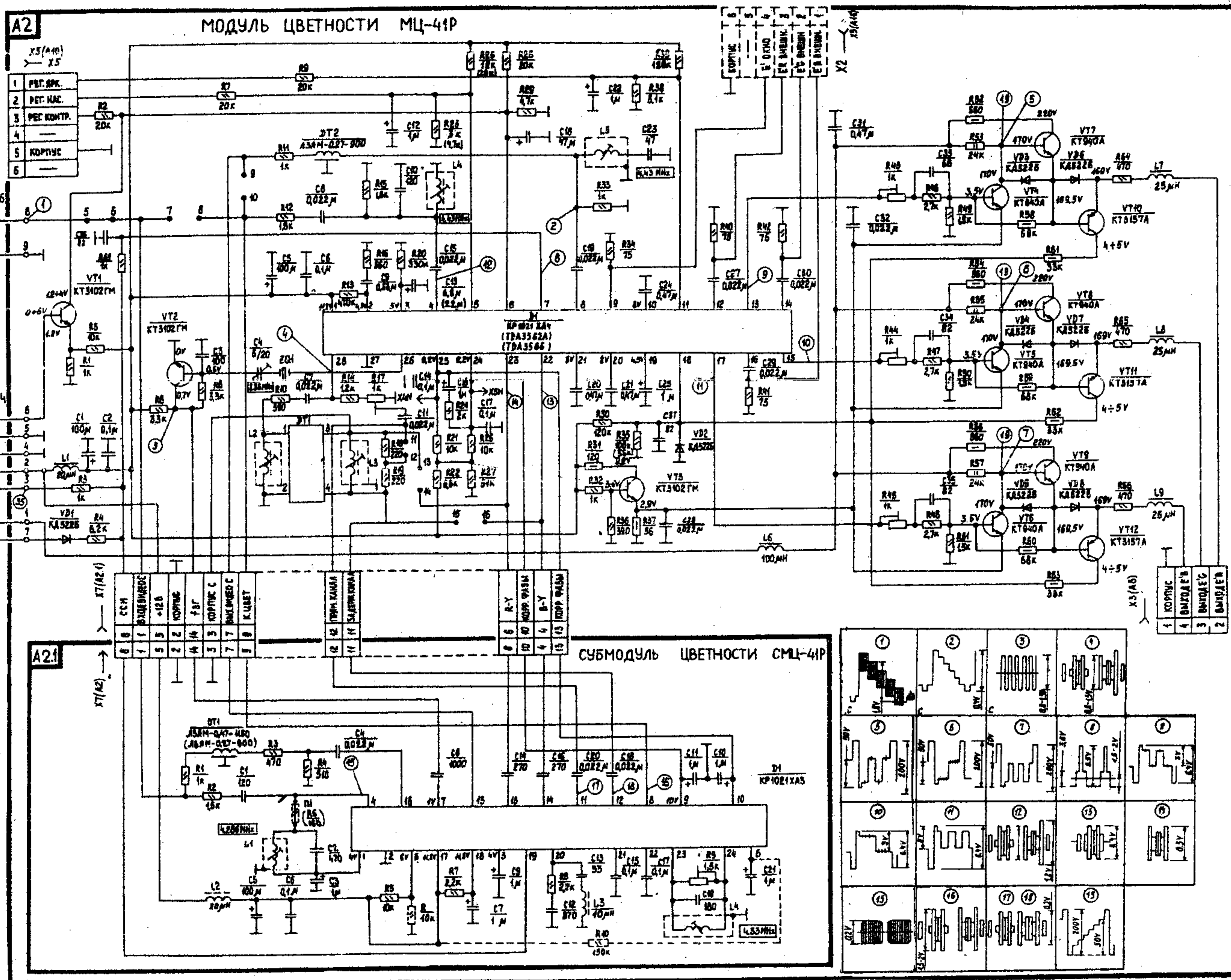
Модули цветности МЦ - 41Р, СМЦ-41Р
