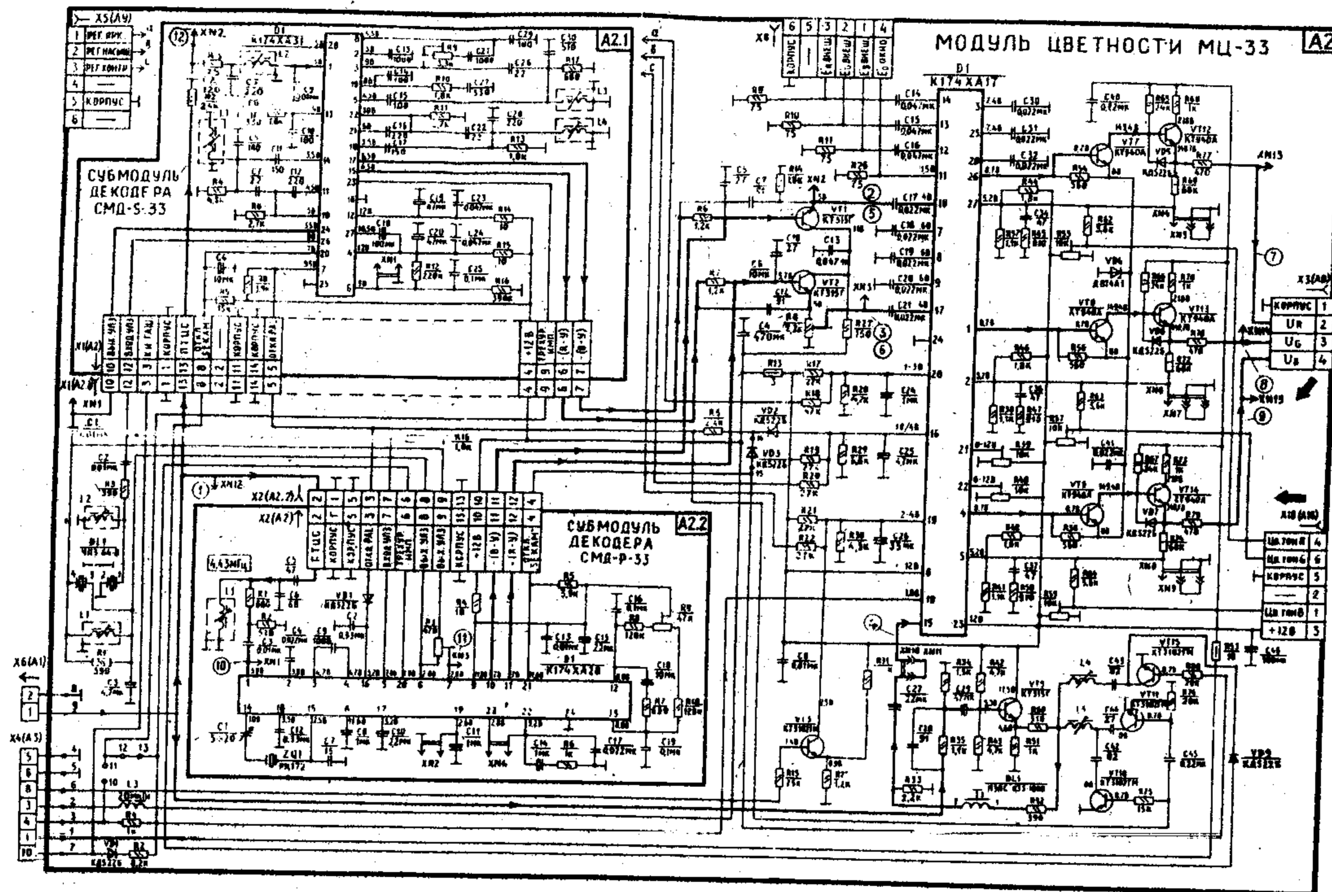
Модули цветности МЦ - 33 (СМД-S-33, СМД-P-33)
