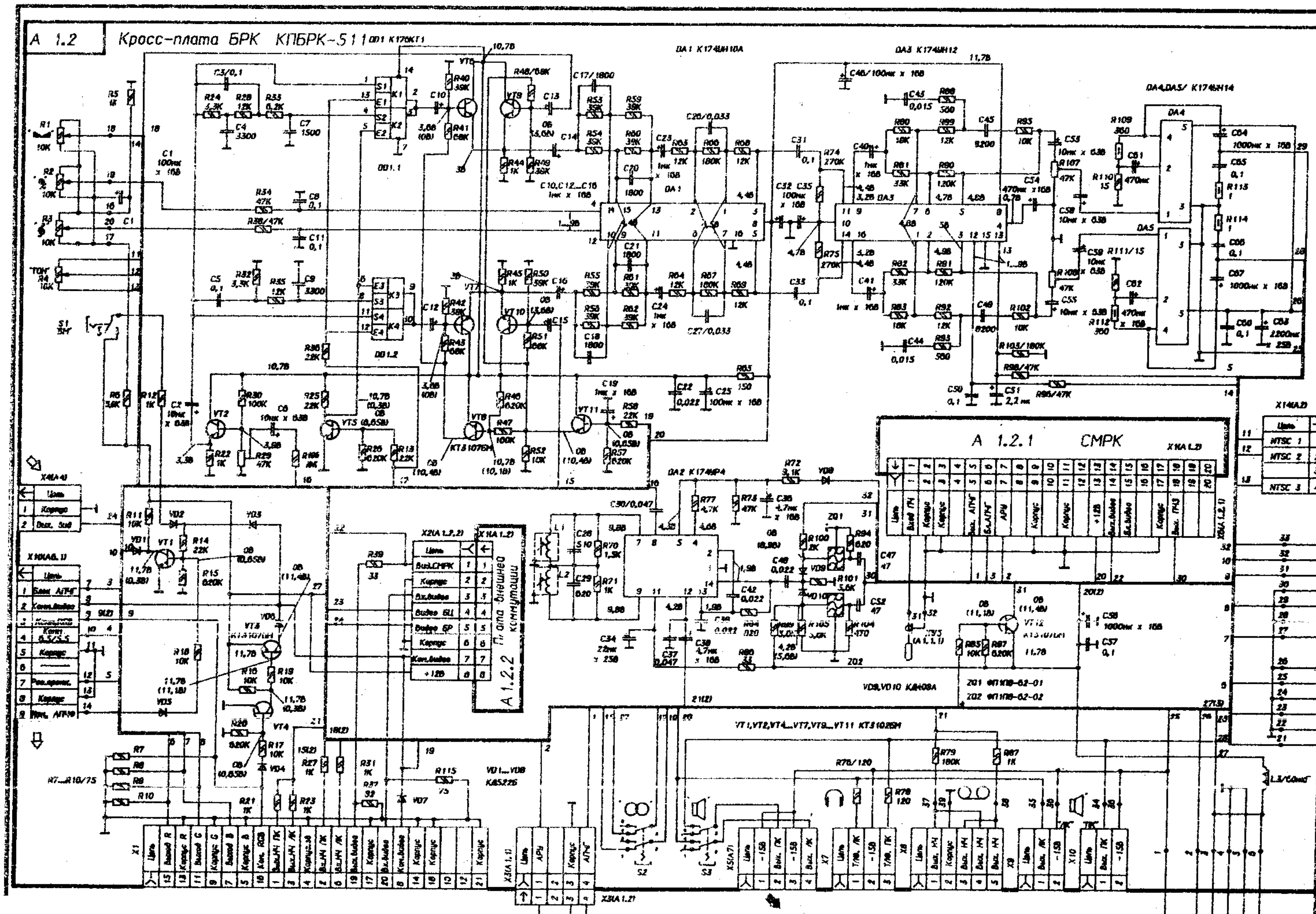
Кросс-плата БРК КП БРК-511(СМРК, ПВК)
