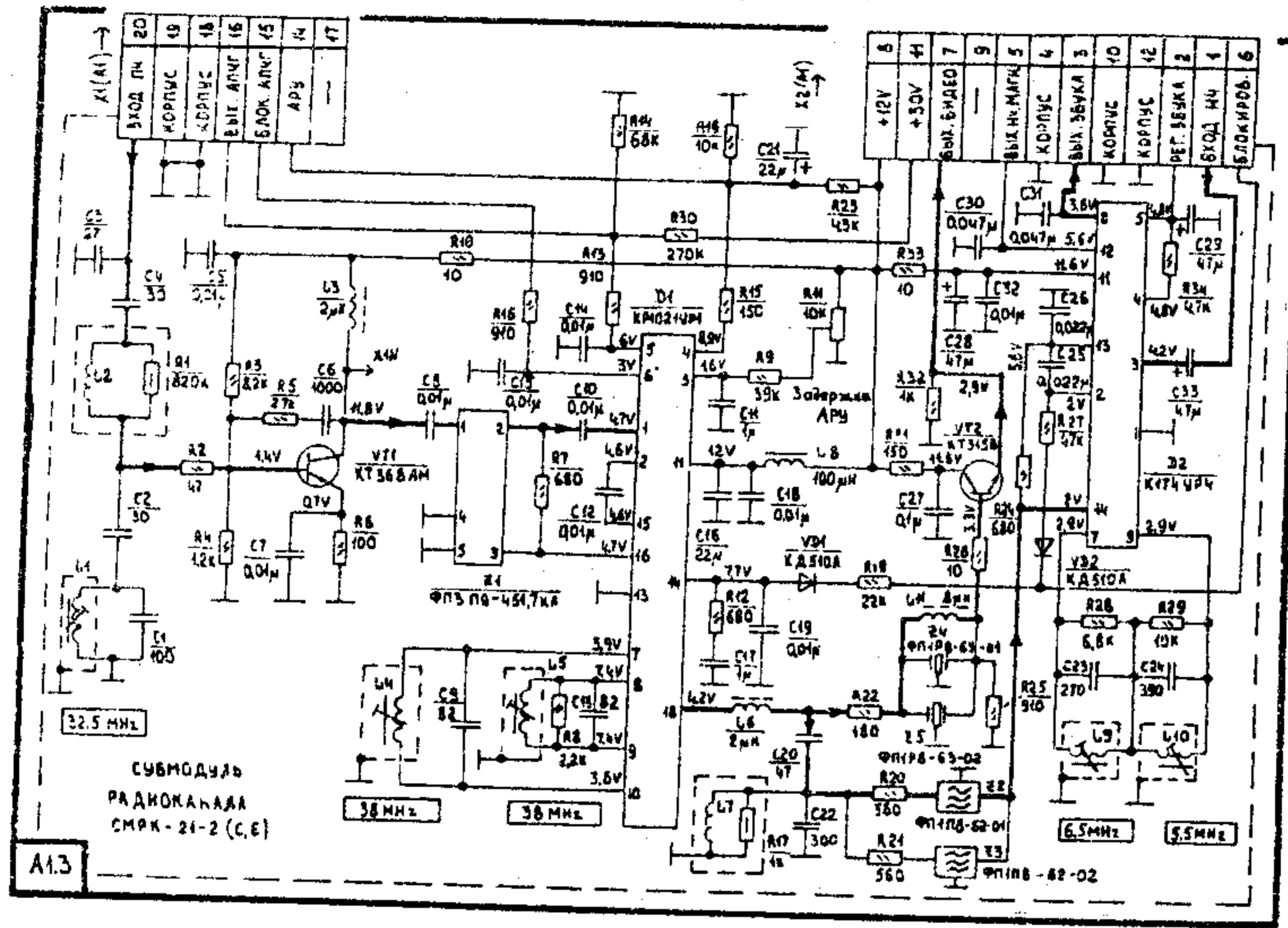
Субмодуль радиоканала СМРК-21-2 (С, Е)
