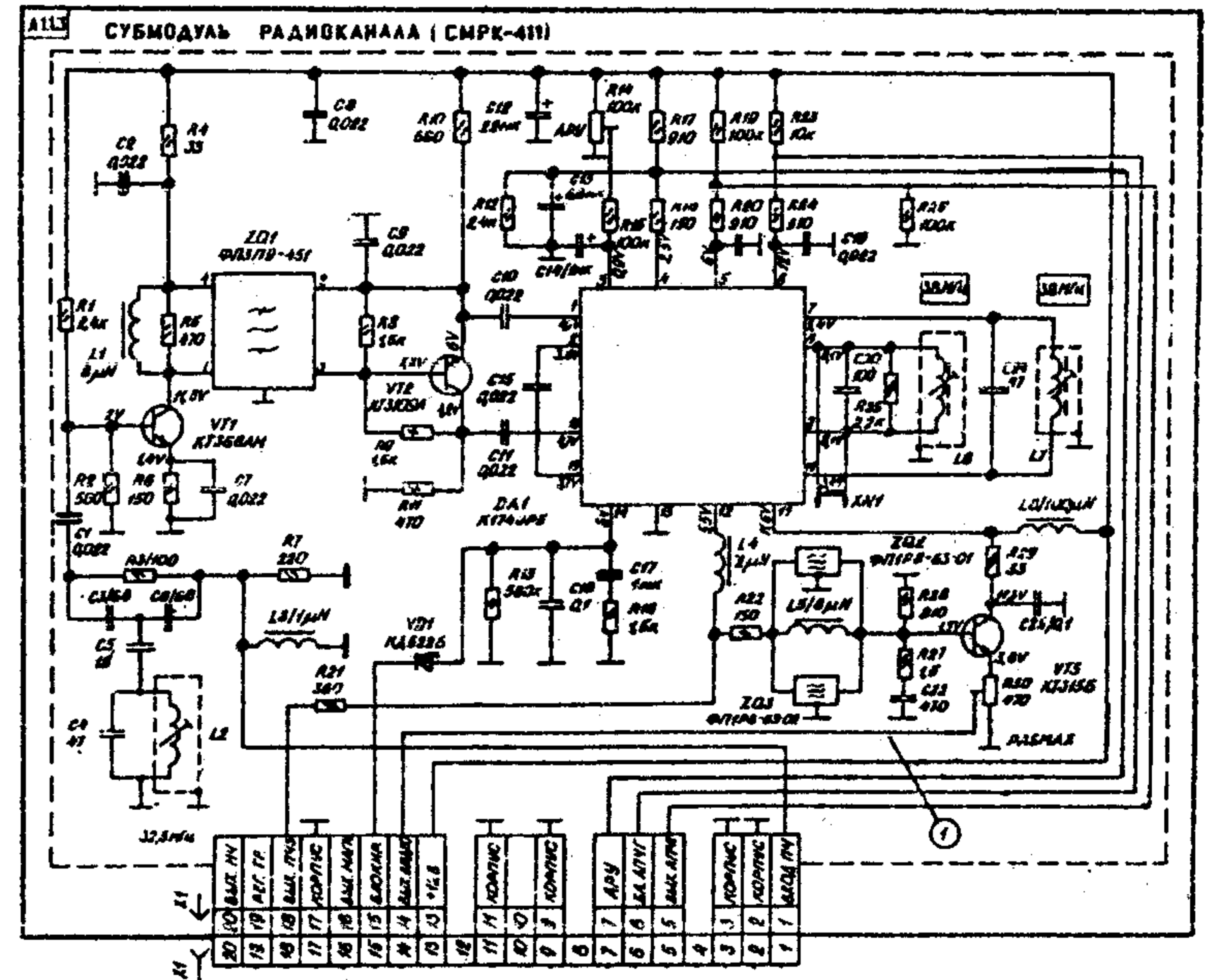
Субмодуль радиоканала СМРК-411
