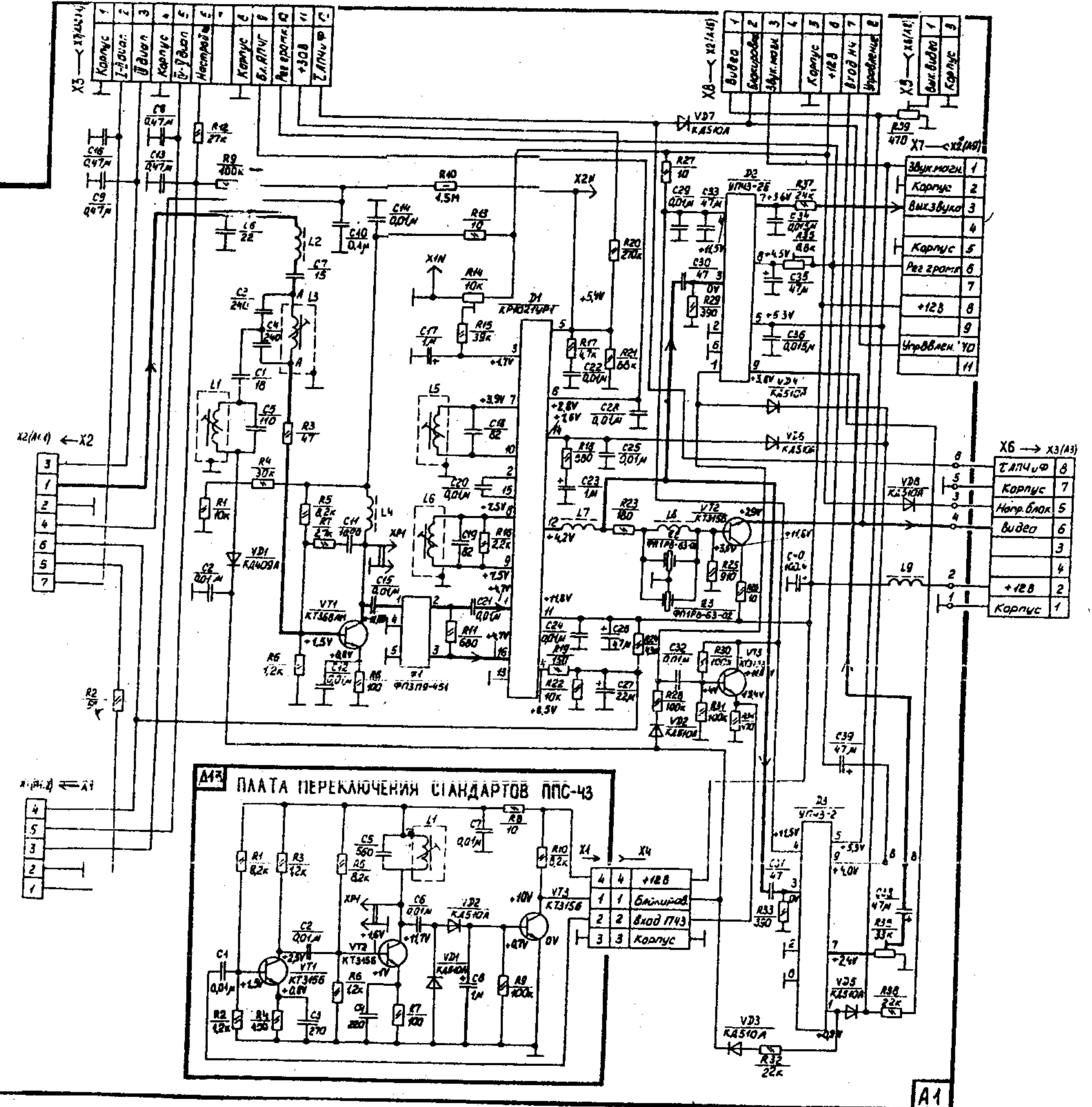
Модуль радиоканала МРК - 43 - 2 (СК-М-24-2С, СК-Д-24С, ППС-43)
