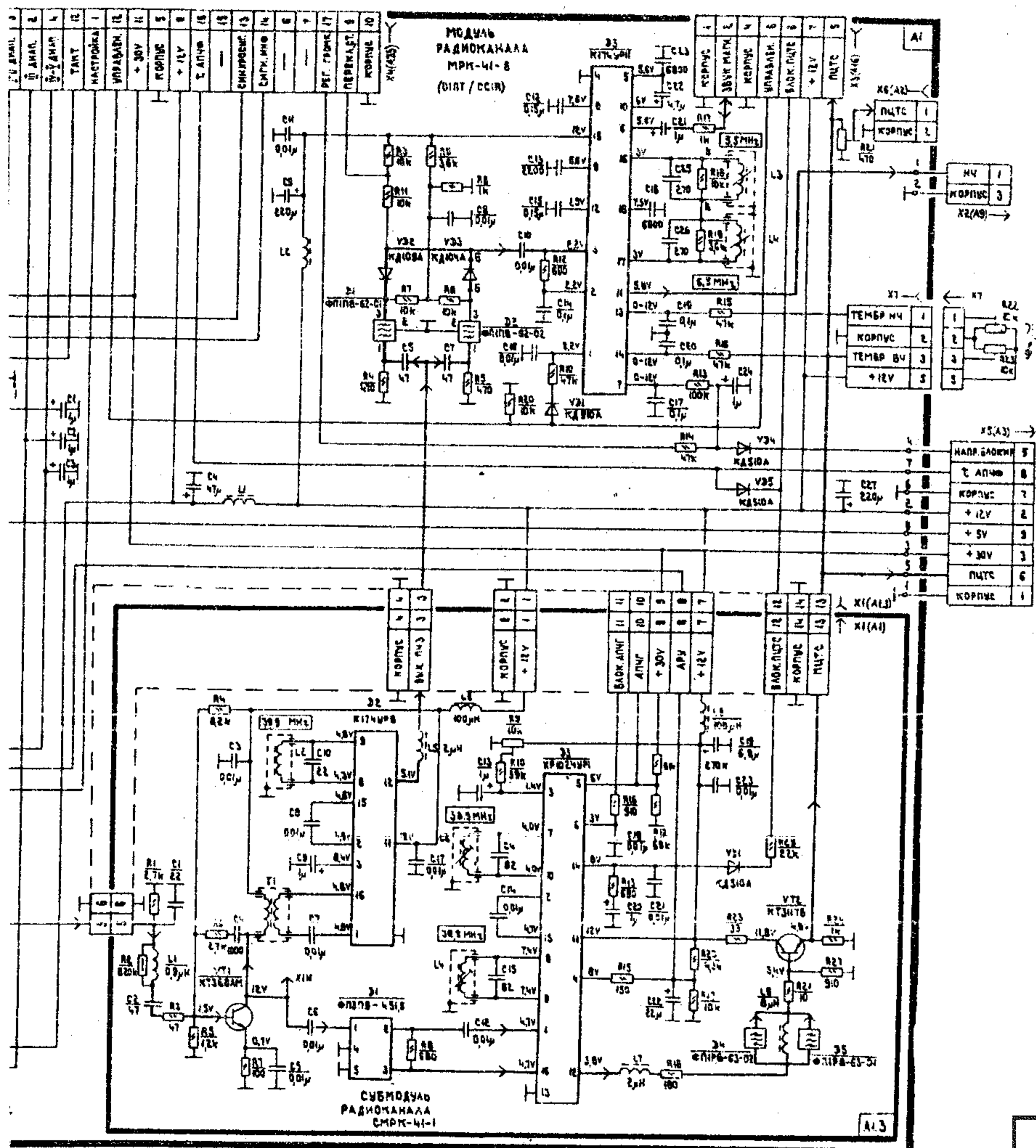
Модуль радиоканала МРК-41-6
