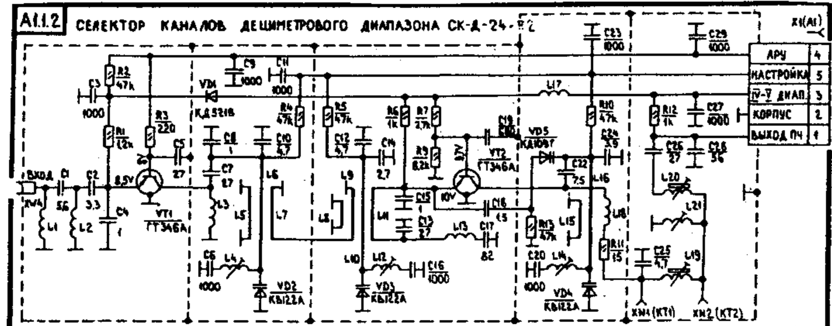
Модуль радиоканала МРК - 2 - 7 РД1 (СК-М-24-2С, СК-Д-24-ЕС2, СМРК - 2- 1Р, УСР-Р, ПО)
