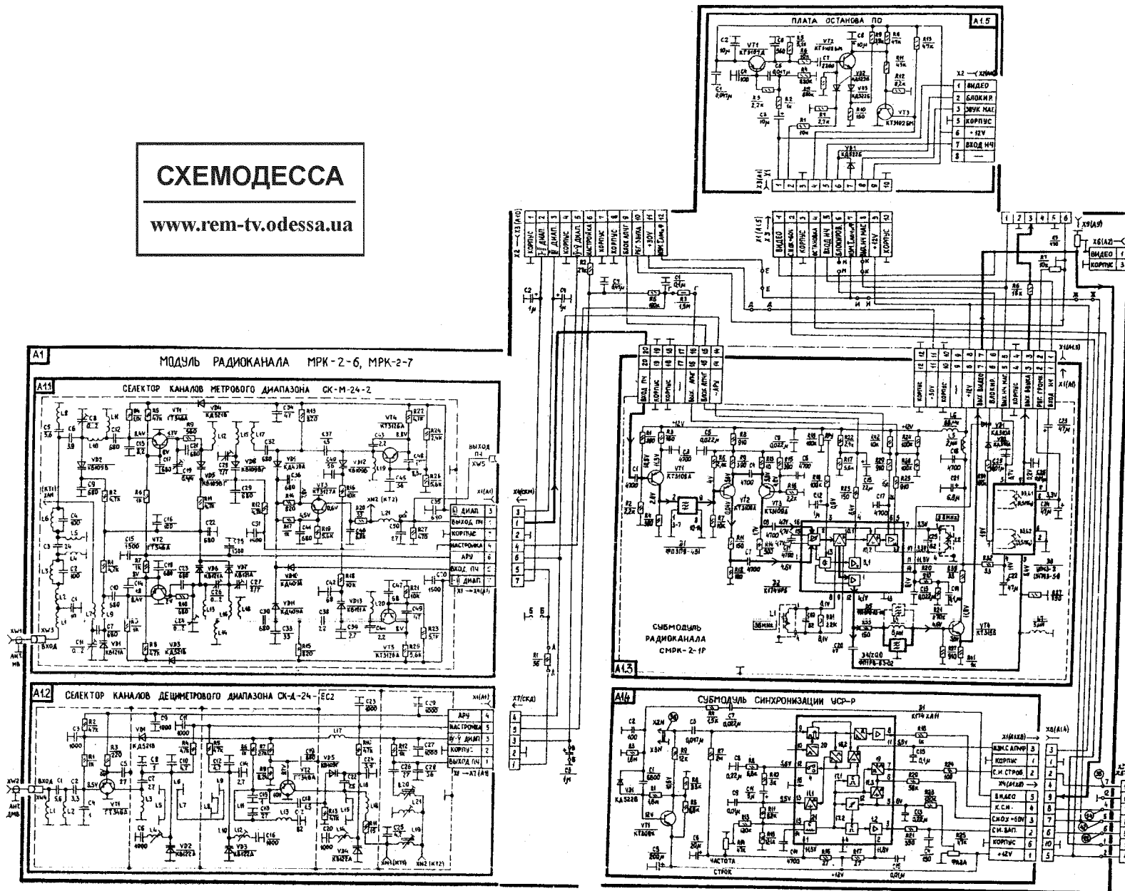
Модуль радиоканала МК-2-6, МК-2-7 (СК -М-24-2, СК-Д-24-ЕС2, СМК-2 - 1Р, УСП-Р, ПО)
