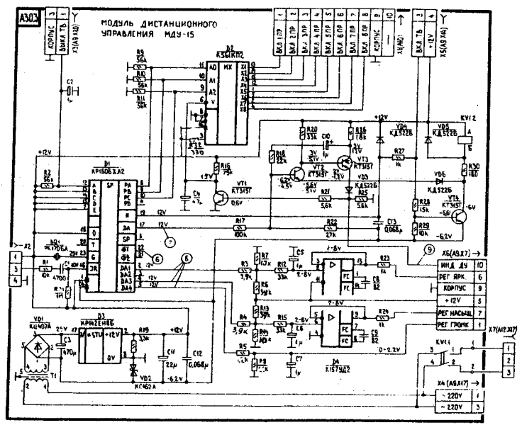
Система дистанционного управления СДУ-4-3 (МДУ -1-3), МДУ-15
