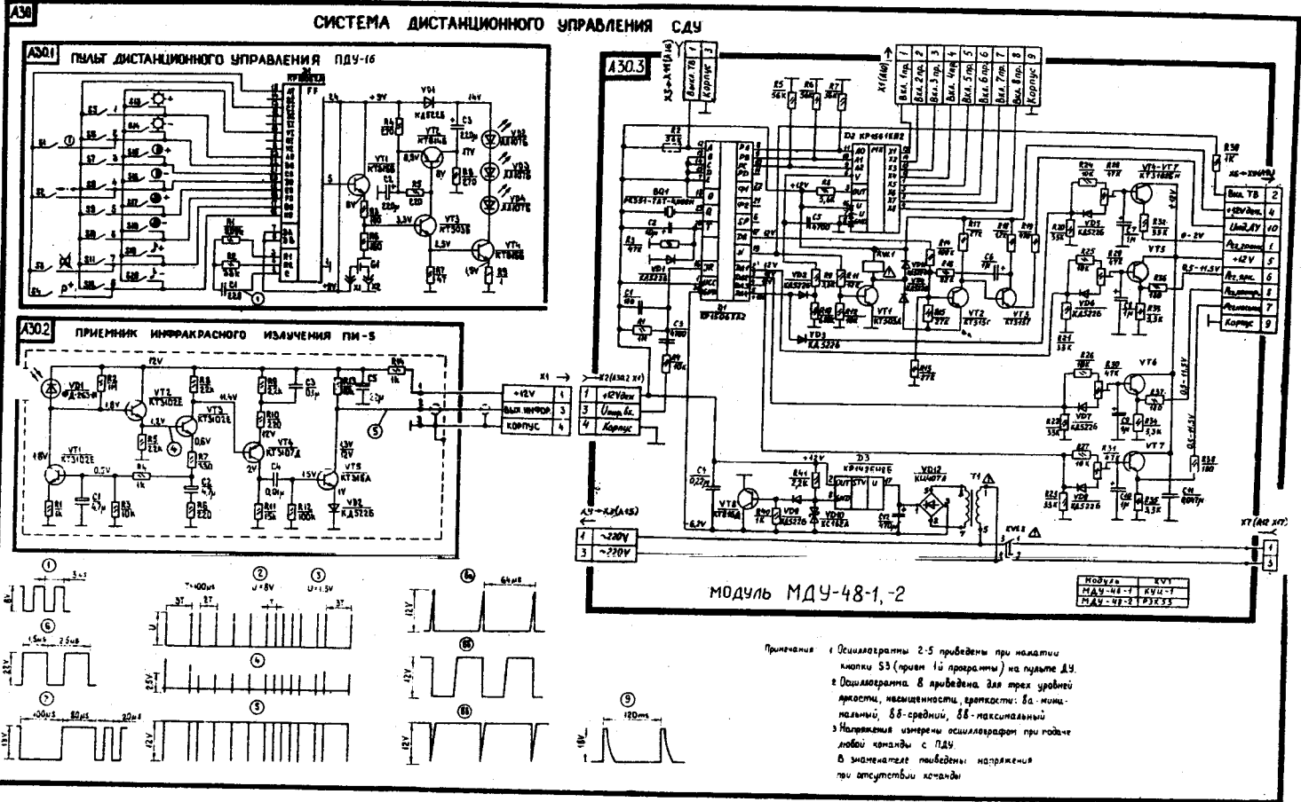
Система дистанционного управления СДУ (ПДУ-16, ПИ-5, МДУ-48-1,2)
