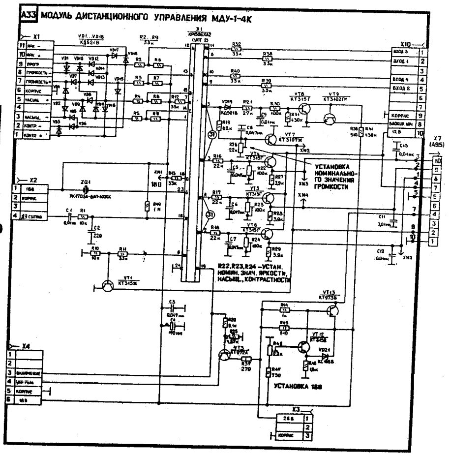
Модуль дистанционного управления МДУ-1-4К
