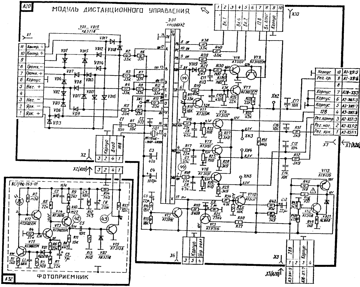
Модуль дистанционного управления МДУ
