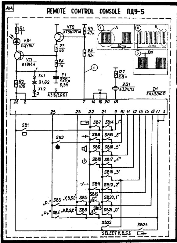
Пульт дистанционного управления ПДУ, ПДУ-2, ПДУ-5, ПДУ-15, ПДУ-16
