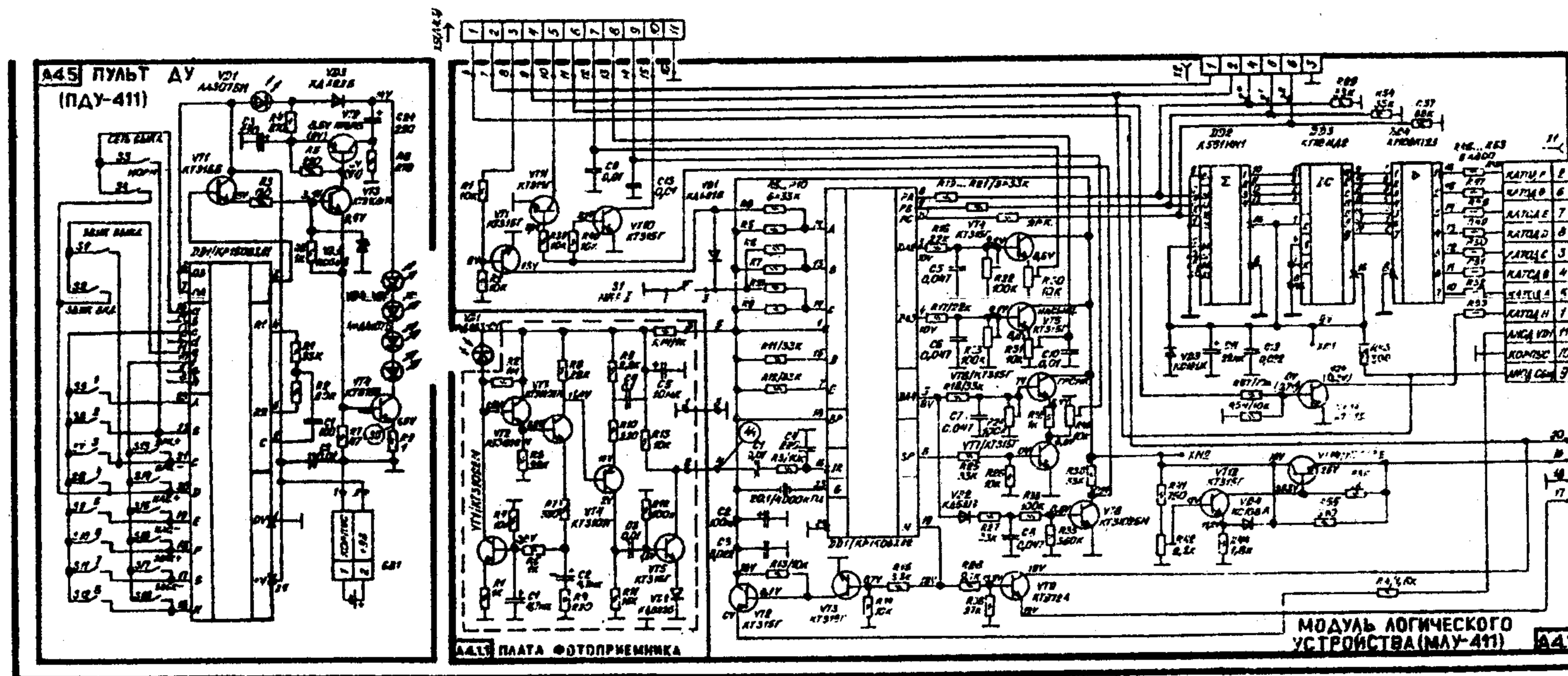
Модуль логического устройства МЛУ-411
