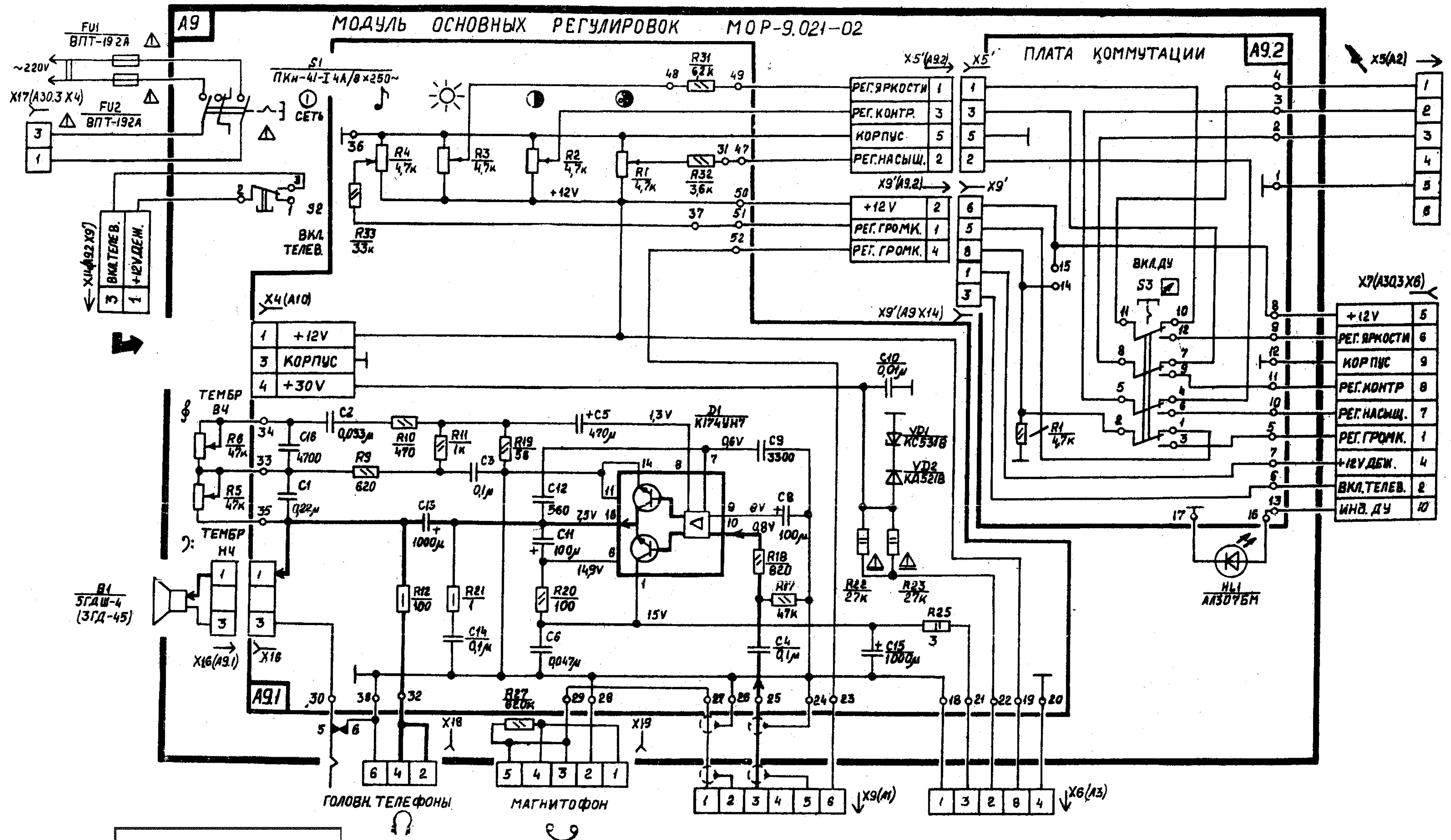
Блоки управления МОР-9, 021-02
