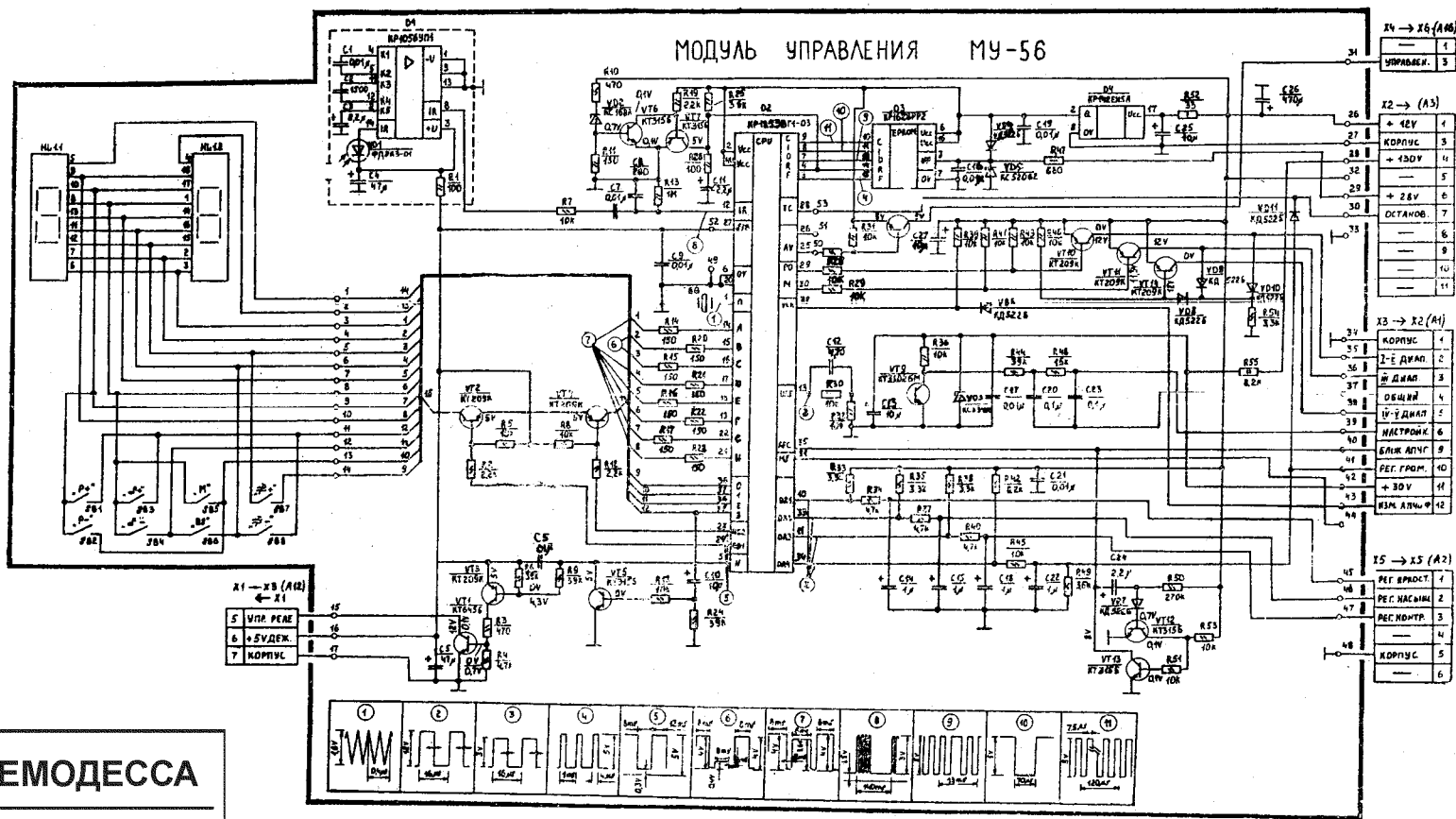
Модуль управления МУ-56
