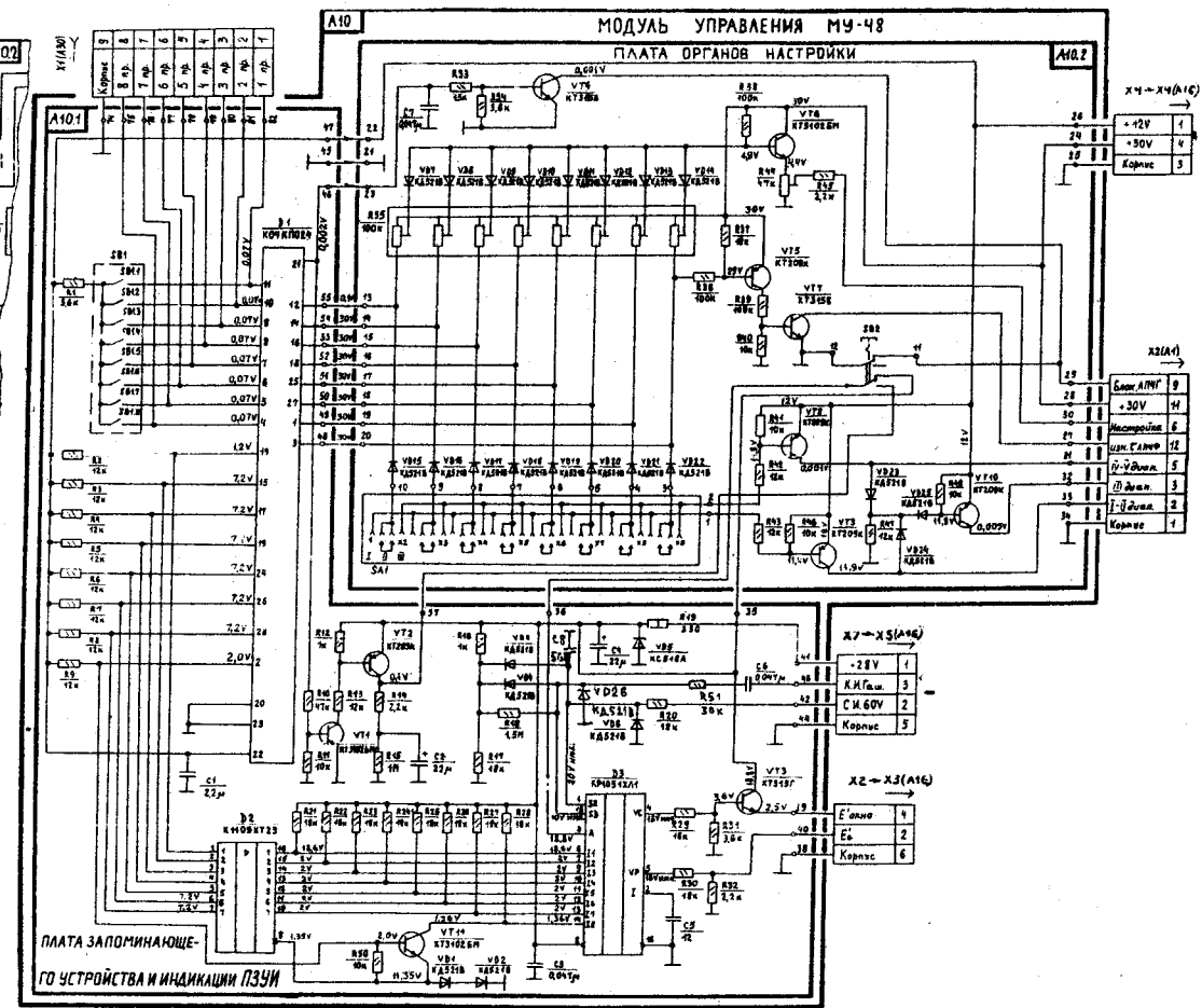
Модуль управления МУ-48
