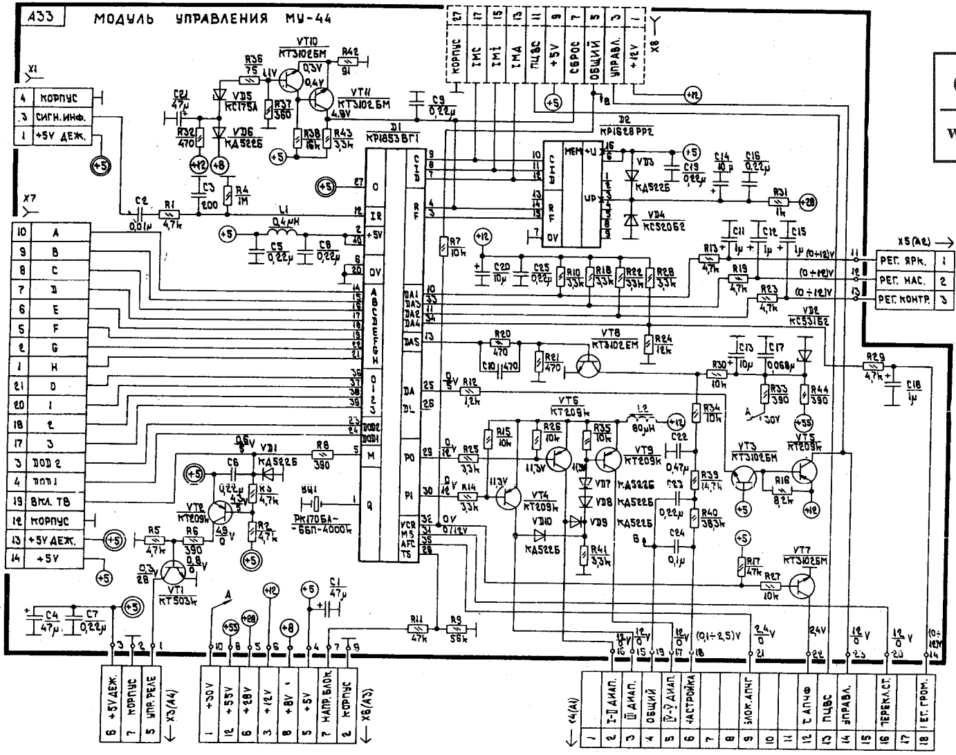
Модуль управления МУ-44
