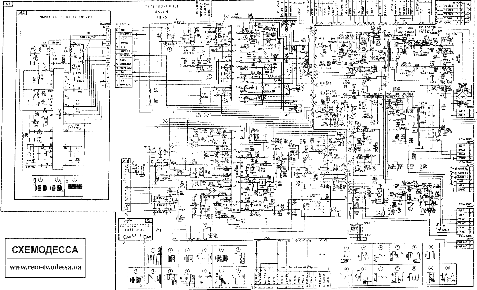
Телевизионное шасси ТШ-5
