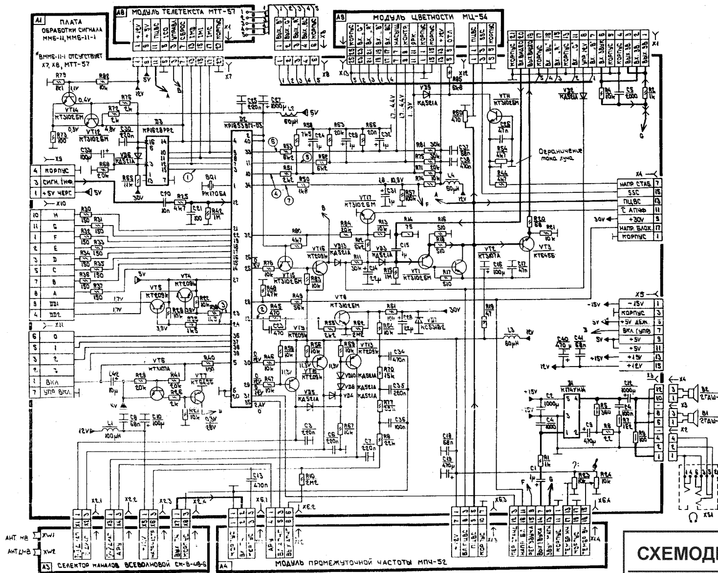
Плата обработки сигнала ММ6-11.
