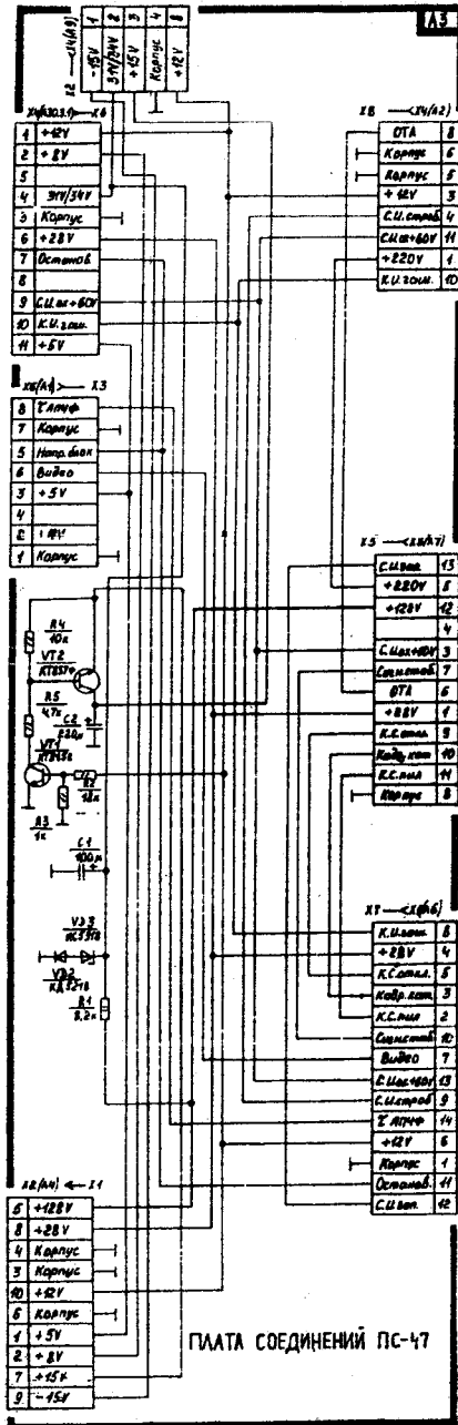
Платы соединения ПС-47, ПС-501, ПС-51
