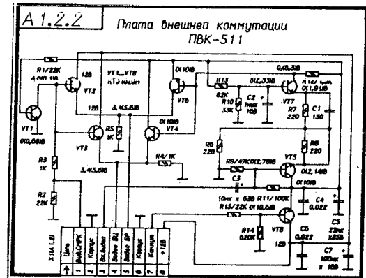
Платы внешней коммутации ПКВ-50, ПКВ-51, ПКВ-52, КП-57, ПКВ-511
