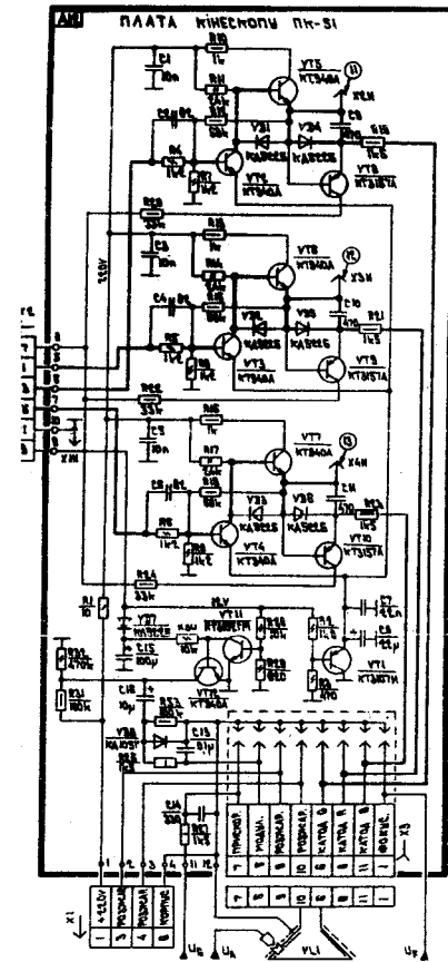
Плата кинескопа ПК-51
