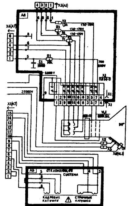
Плата кинескопа ПК - 45
