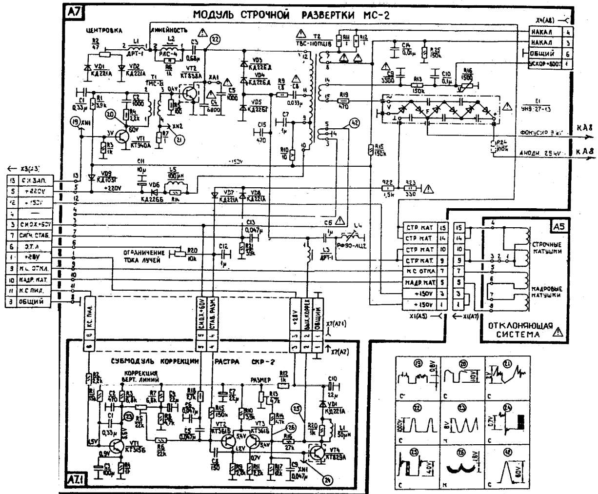
Модули строчной развертки МС-2
