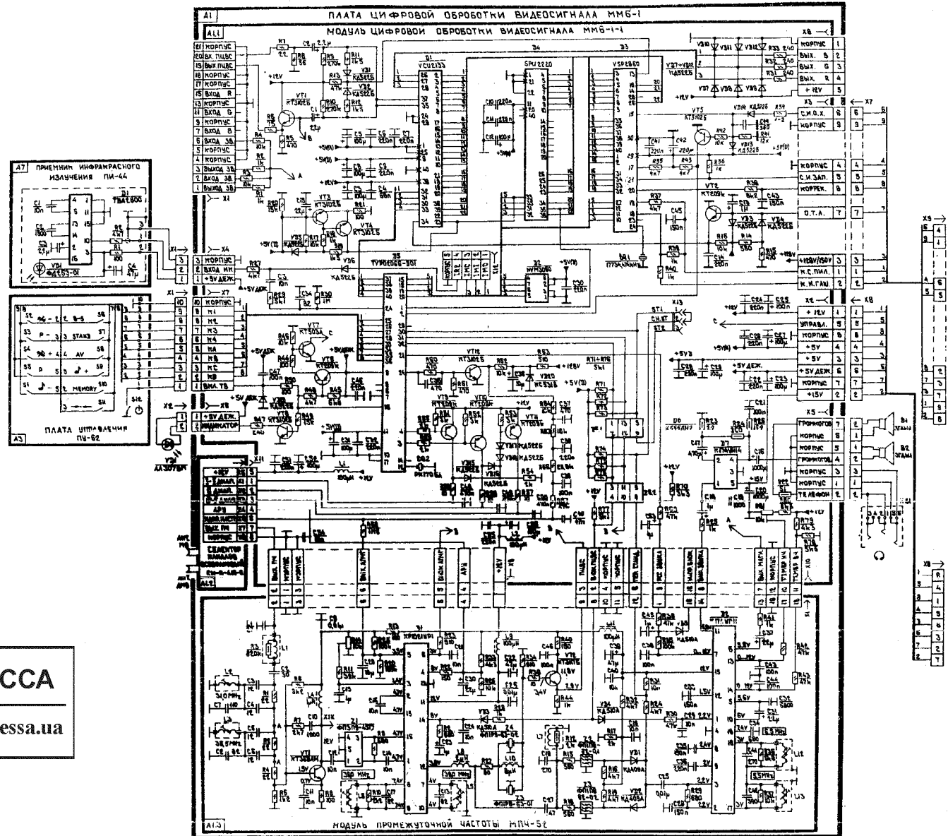
Плата цифровой обработки сигнала ММ6-1.
