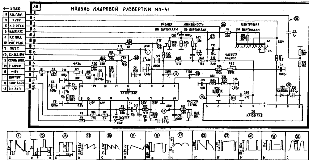
Модуль кадровой развертки, МК-41
