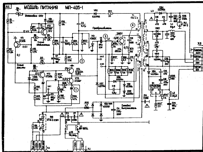
Модуль питания МП - 405 - 1
