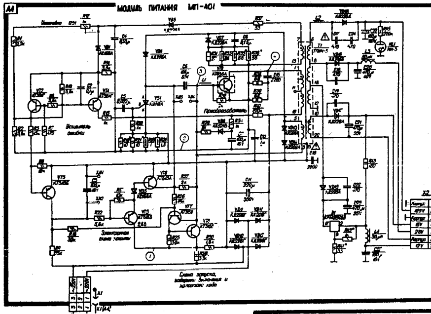
Модуль питания МП - 401
