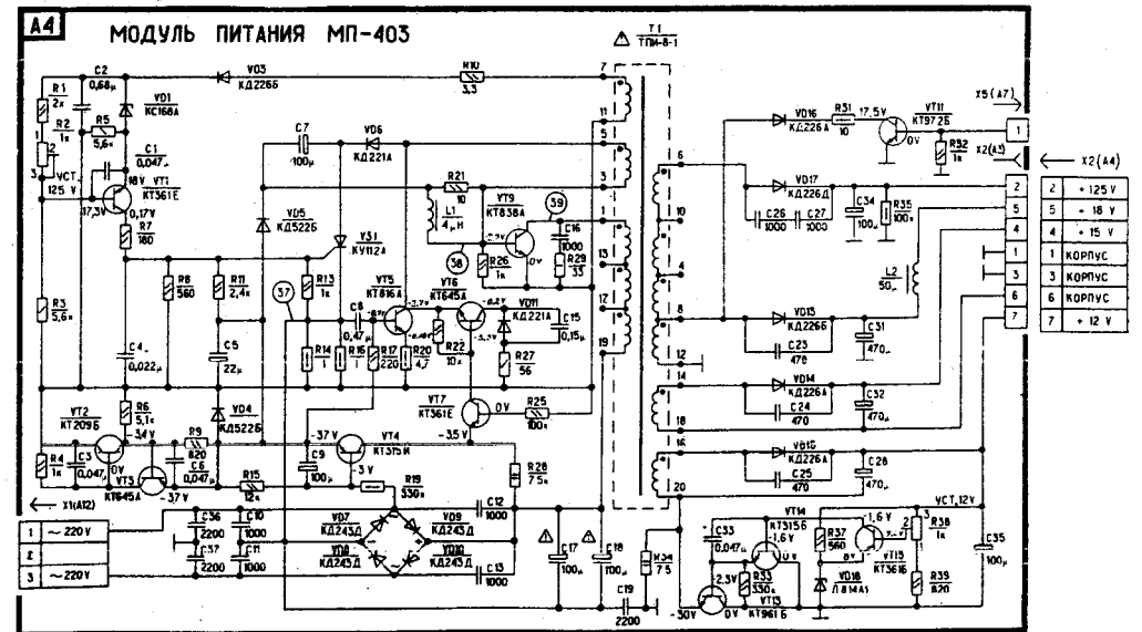
Модуль питания МП-403
